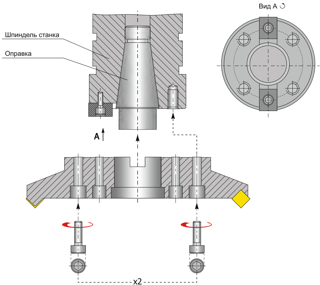
Пример крепления
