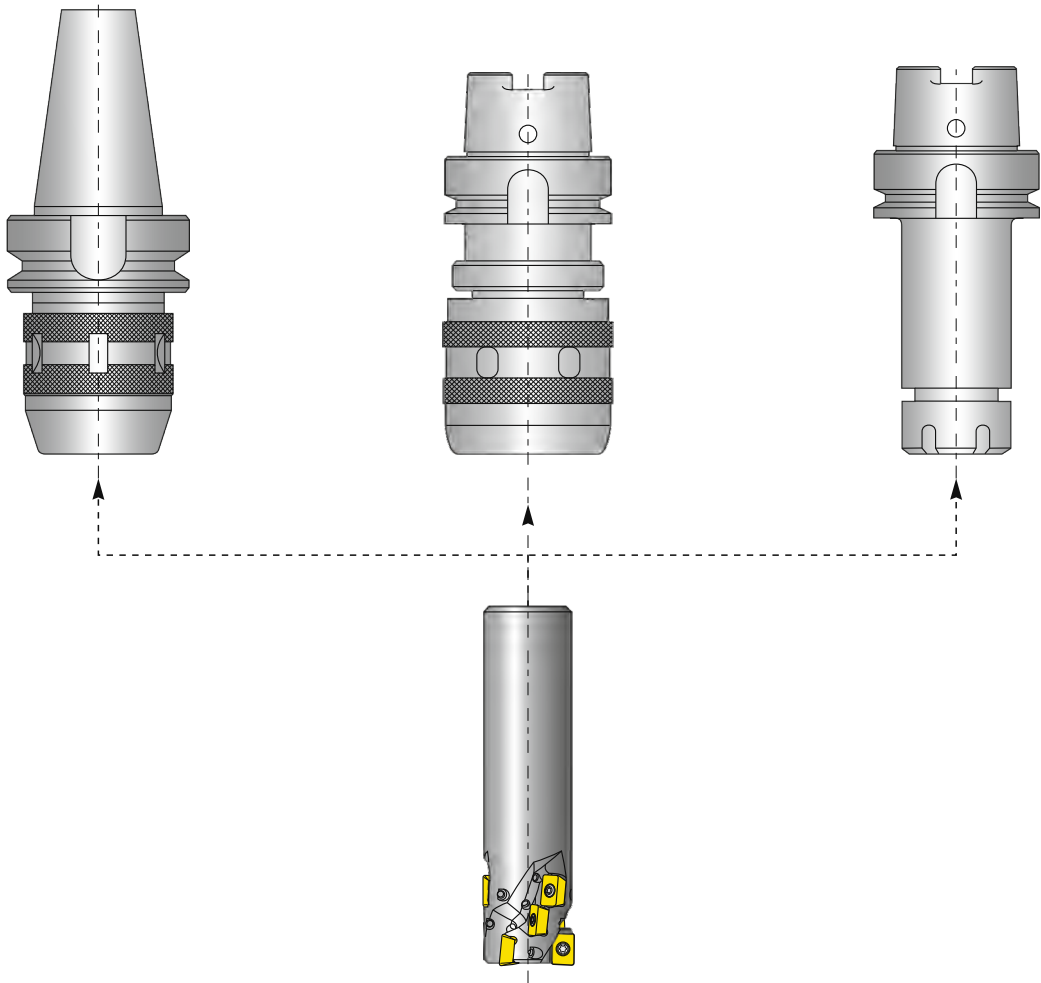
Пример крепления
